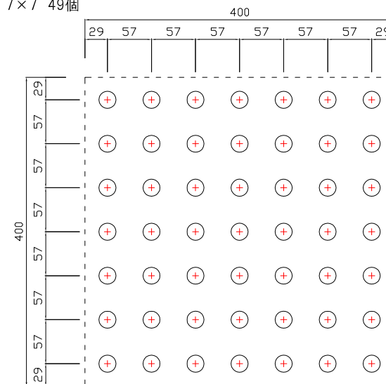
点字鋇基本配列(JIS)400角の場合 7×7 49個
