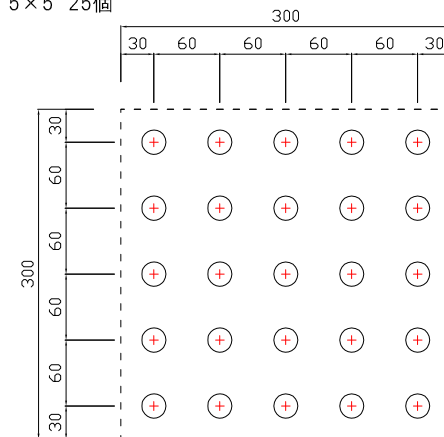
点字鋇基本配列(JIS)300角の場合 5×5 25個
