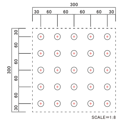
点字鋏基本配列(JIS)300角の場合 5×5 25個
