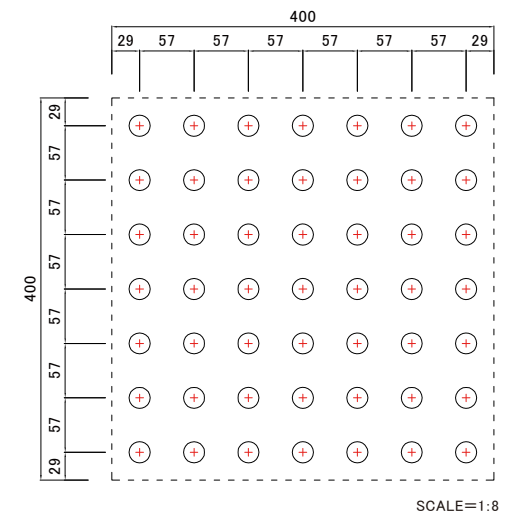
点字鋏基本配列(JIS)400角の場合 7×7 49個
