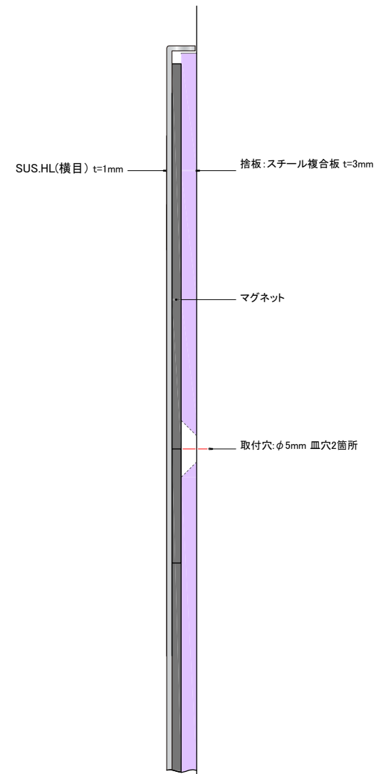
A-A SCALE 1:1
