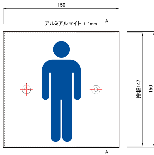
アルミアルマイト BOX型 6mm 捨板付(マグネット仕様) 表示: カッティングシート貼り
