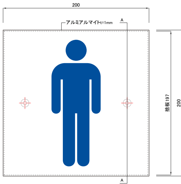
アルミアルマイトBOX型 6mm 捨板付 (マグネット仕様) 表示: カuttingシート貼り
